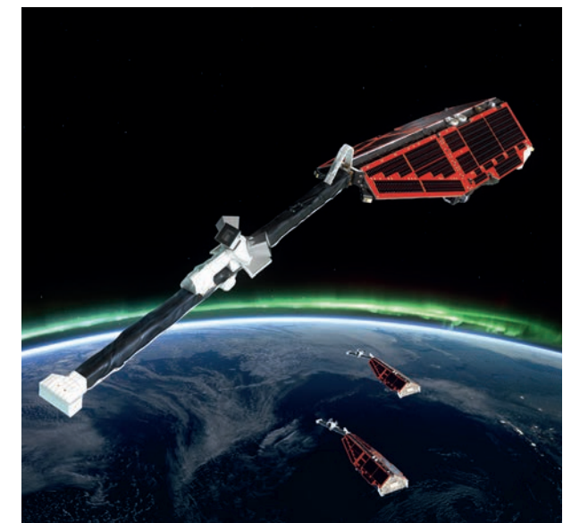
Rechts: Schematische Abbildung der für die Studie benutzte Swarm-Satelliten. Im Hintergrund die teilweise ionisierte Erdatmosphäre. Abb.: https://earth.esa.int/eogateway/missions/swarm
