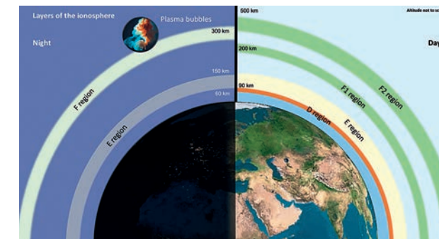
Schematische Darstellung der Atmosphärenschichten, einschließlich der kreisförmig hervorgehobenen Gebiete, in denen die Plasmablasen vorkommen. Abbildung: Siddiqui, IAP
